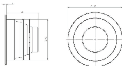
D10-B2-6w-12w Size 10 Bevel IP54
