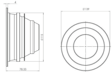
D12-B2-6w-12w-18w Size 12 Bevel IP54
